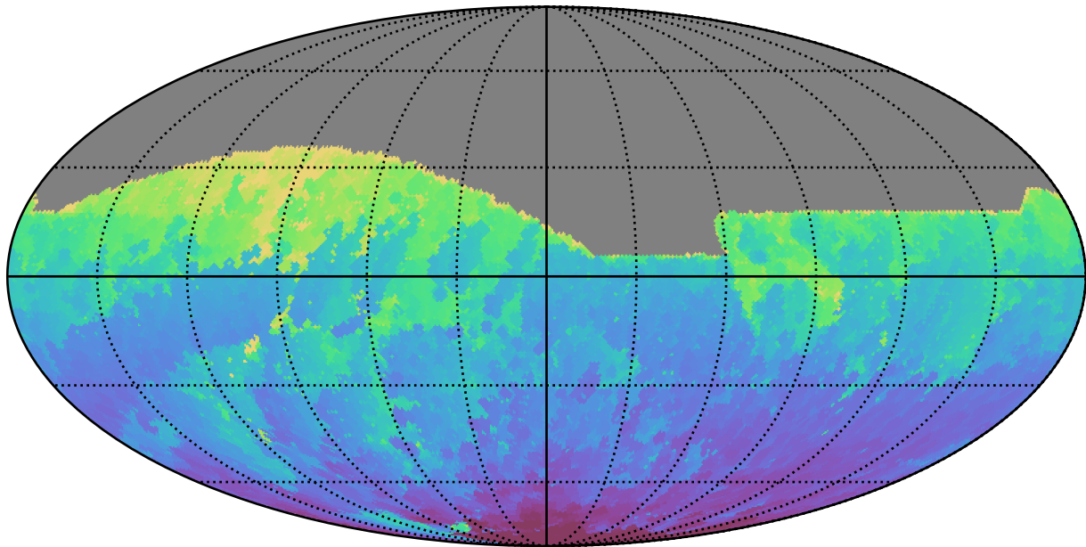
extra_ss_neo4_v3.4_10yrs All sky z band: Min HA
