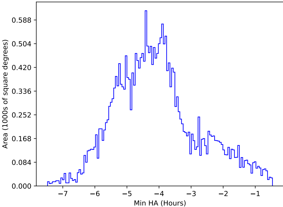
extra_ss_neo4_v3.4_10yrs All sky z band: Min HA
