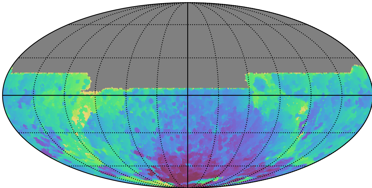
extra_ss_neo4_v3.4_10yrs All sky y band: Min HA
