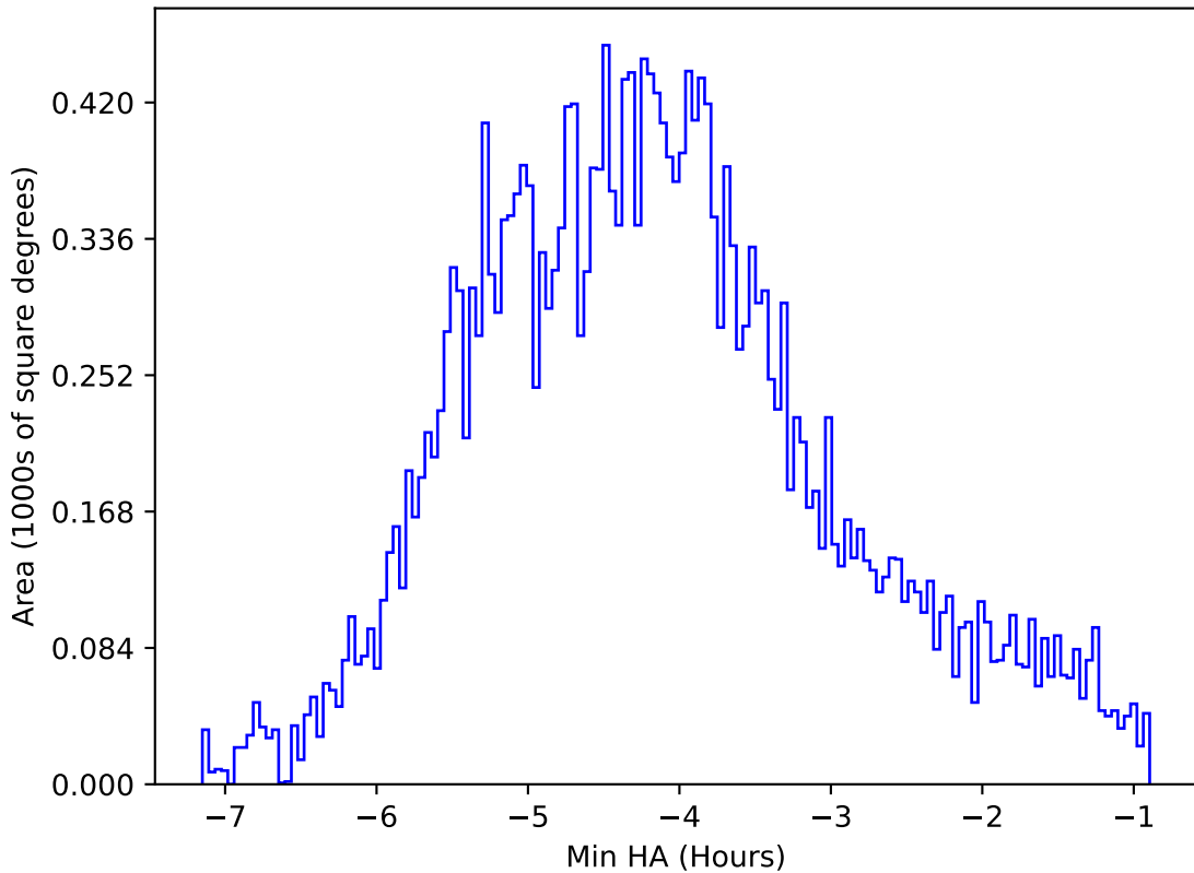
extra_ss_neo4_v3.4_10yrs All sky r band: Min HA
