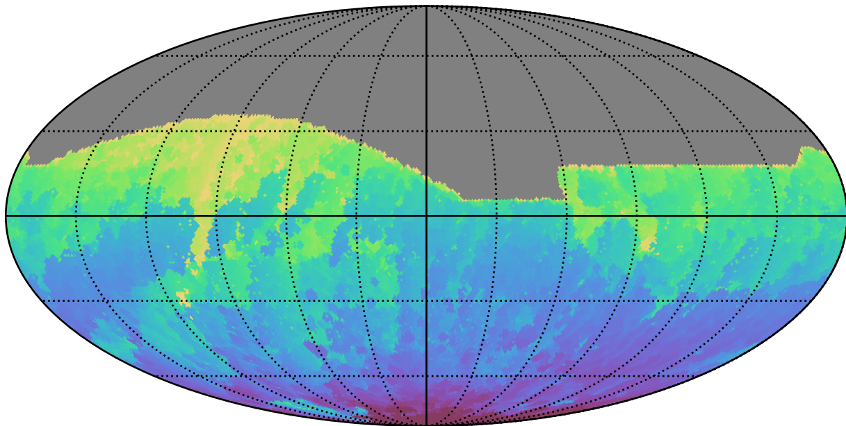
extra_ss_neo4_v3.4_10yrs All sky i band: Min HA
