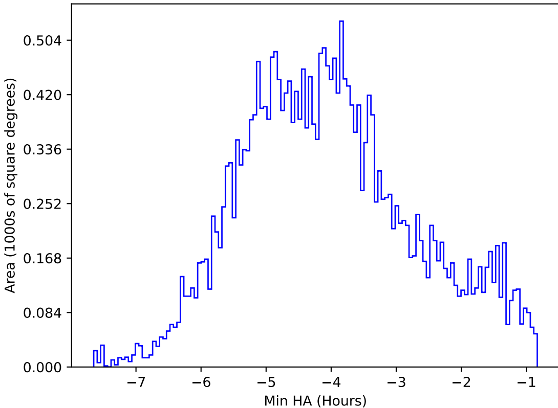
extra_ss_neo4_v3.4_10yrs All sky i band: Min HA
