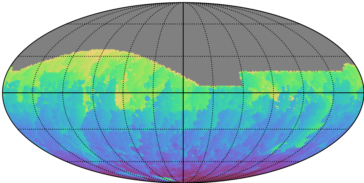
extra_ss_neo4_v3.4_10yrs All sky g band: Min HA
