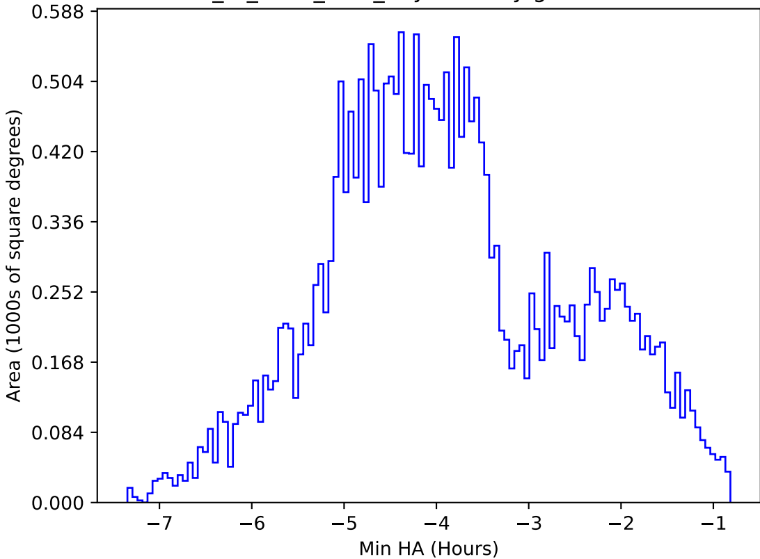
extra_ss_neo4_v3.4_10yrs All sky g band: Min HA
