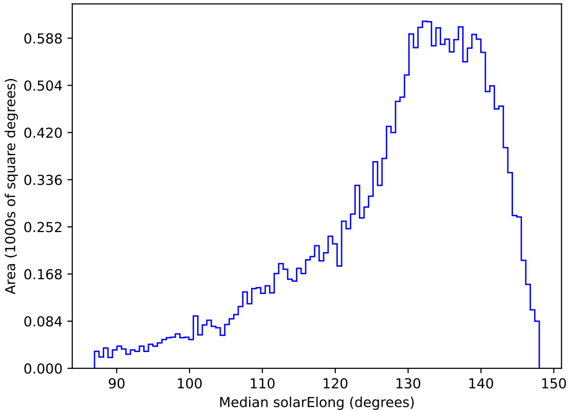
extra_ss_neo4_v3.4_10yrs All sky y band: Median solarElong
