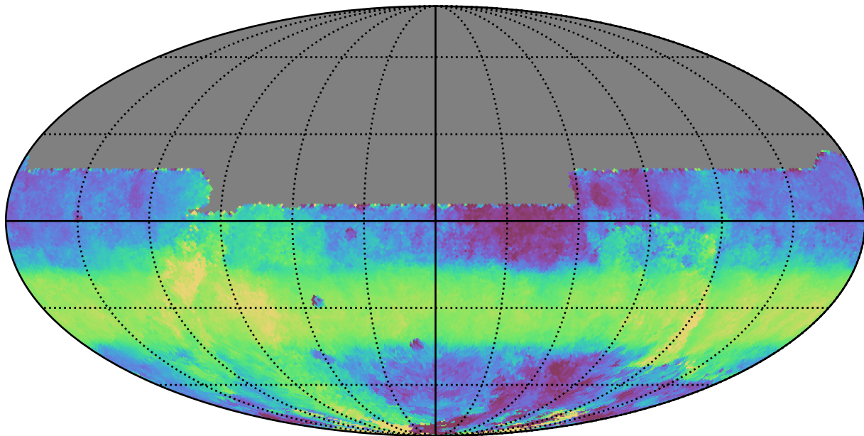
extra_ss_neo4_v3.4_10yrs All sky y band: Median HA
