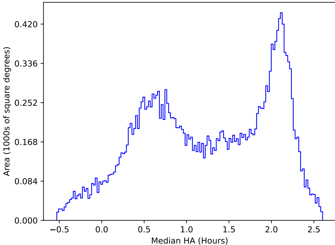
extra_ss_neo4_v3.4_10yrs All sky y band: Median HA
