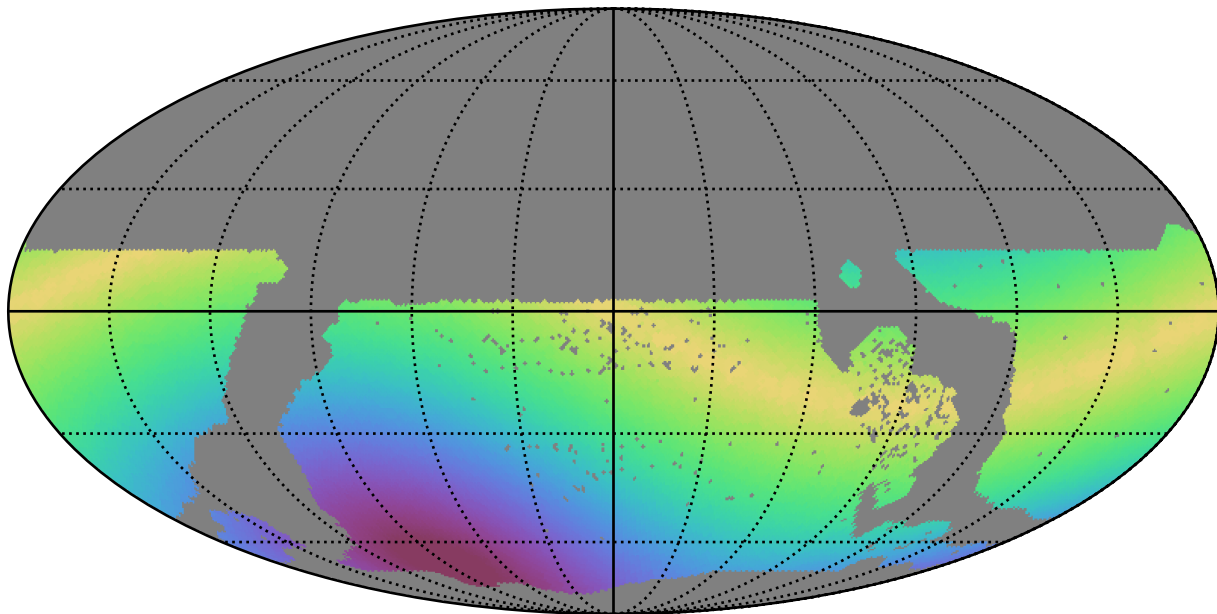
extra_ss_neo4_v3.4_10yrs WFD y band: Max solarElong
