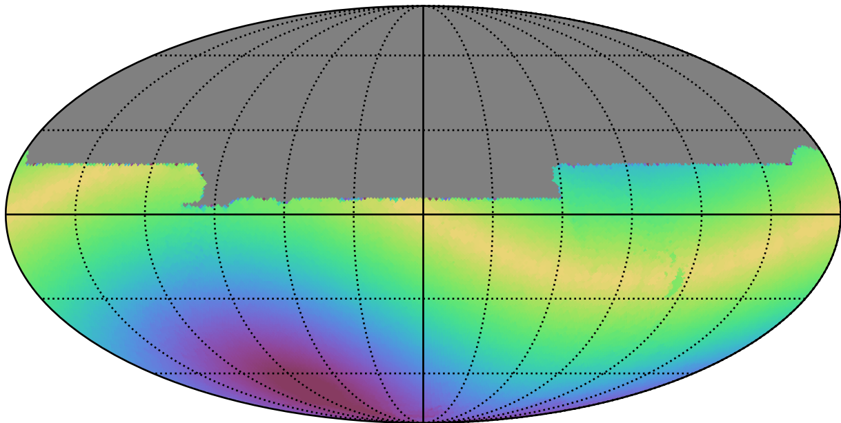
extra_ss_neo4_v3.4_10yrs All sky y band: Max solarElong
