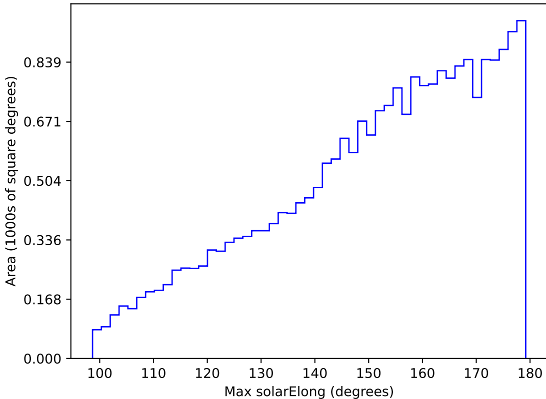
extra_ss_neo4_v3.4_10yrs All sky y band: Max solarElong
