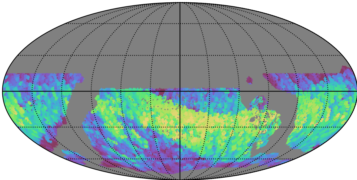
extra_ss_neo4_v3.4_10yrs WFD z band: Max normairmass
