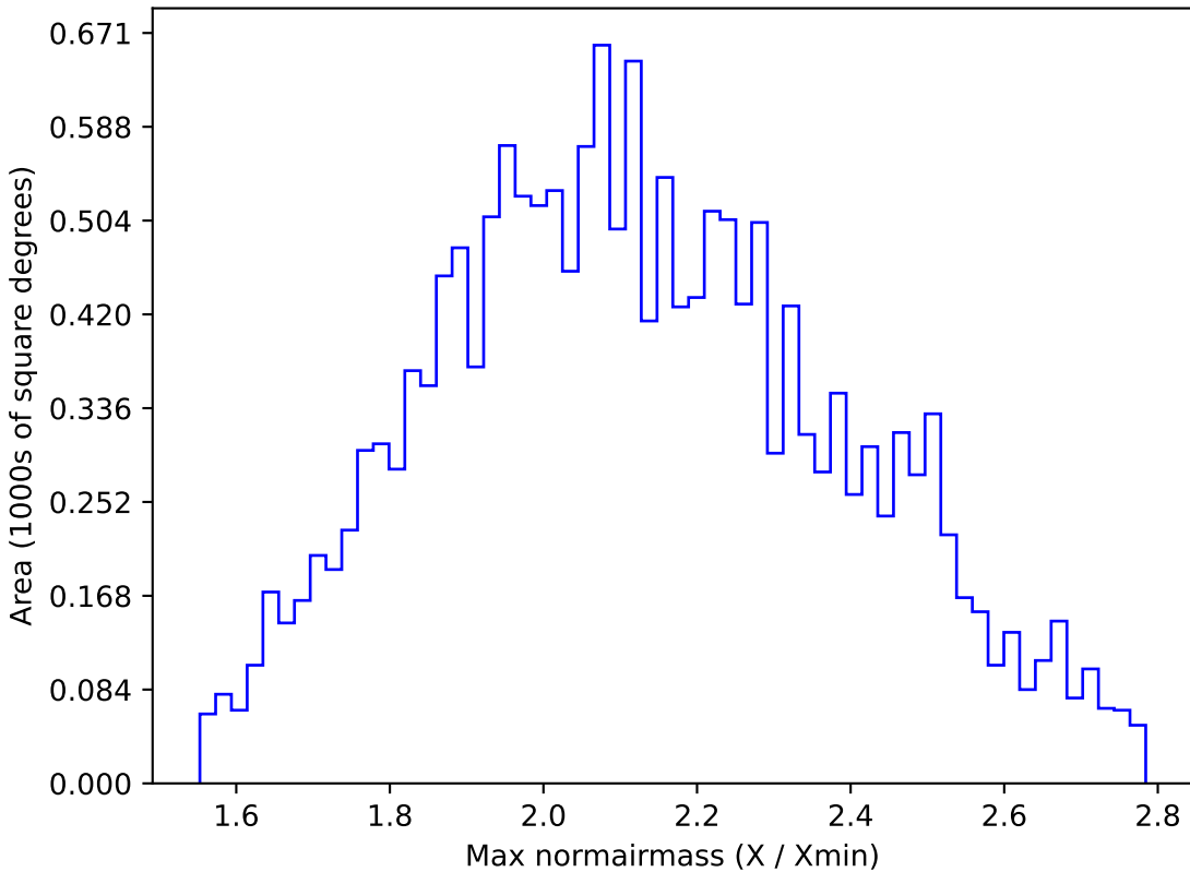
extra_ss_neo4_v3.4_10yrs WFD y band: Max normairmass
