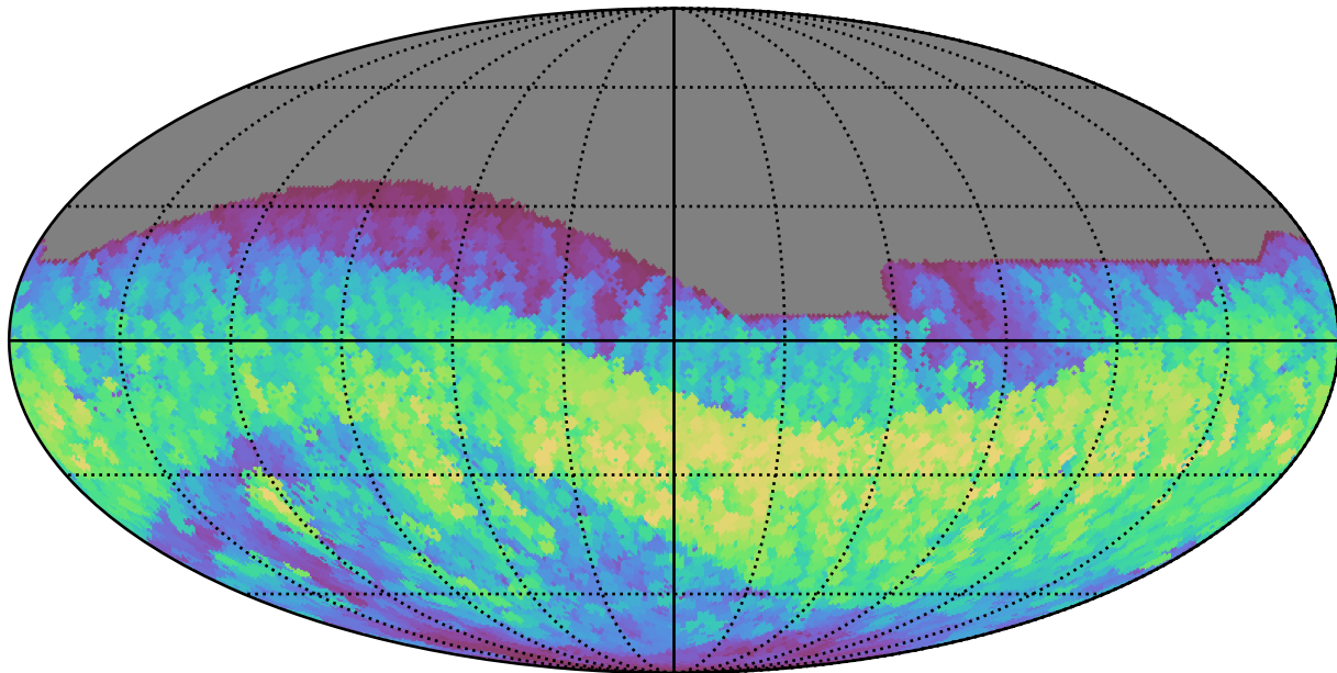
extra_ss_neo4_v3.4_10yrs All sky z band: Max normairmass
