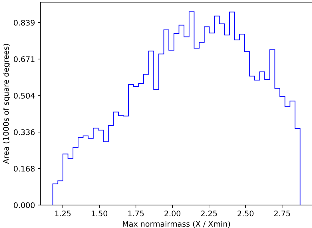
extra_ss_neo4_v3.4_10yrs All sky z band: Max normairmass
