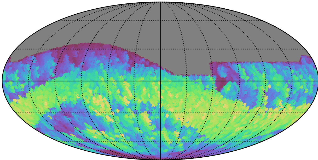
extra_ss_neo4_v3.4_10yrs All sky r band: Max normairmass
