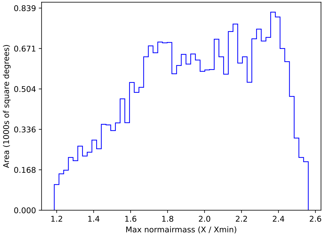
extra_ss_neo4_v3.4_10yrs All sky r band: Max normairmass
