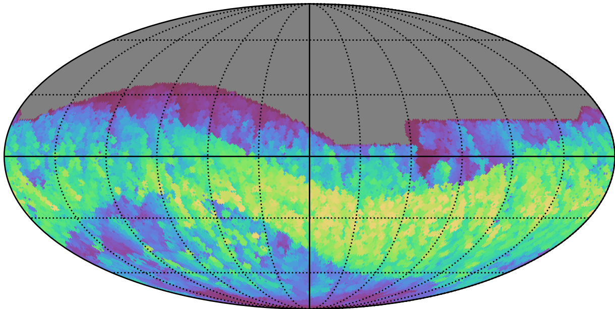
extra_ss_neo4_v3.4_10yrs All sky i band: Max normairmass
