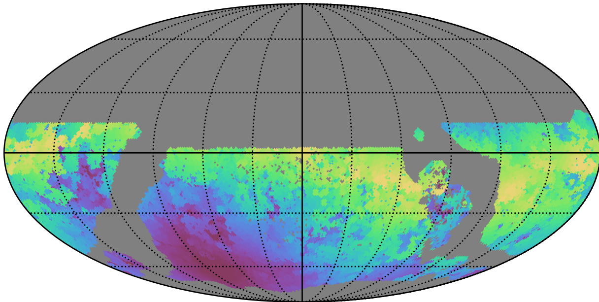
extra_ss_neo4_v3.4_10yrs WFD y band: Max moonDistance
