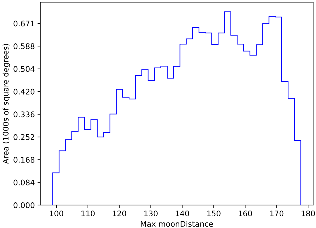
extra_ss_neo4_v3.4_10yrs WFD y band: Max moonDistance
