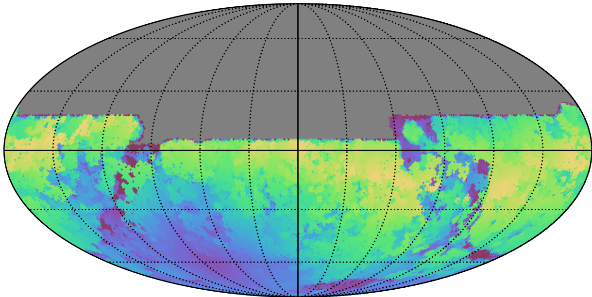
extra_ss_neo4_v3.4_10yrs All sky y band: Max moonDistance
