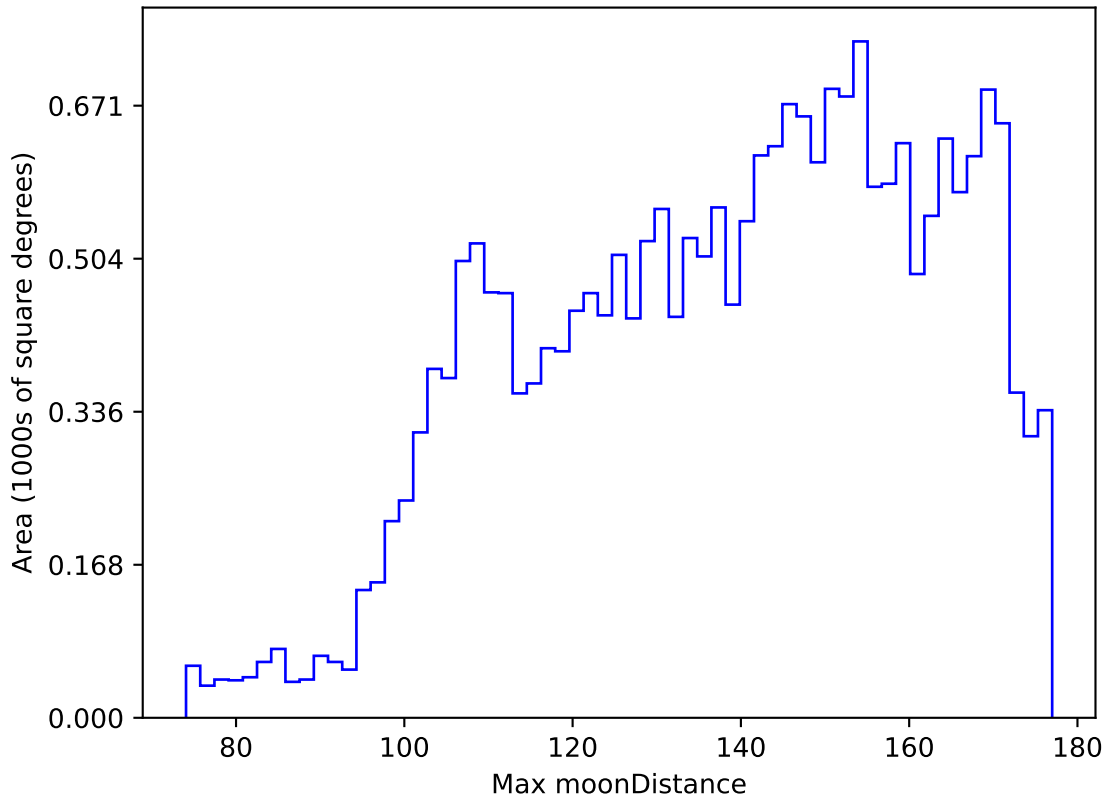
extra_ss_neo4_v3.4_10yrs All sky y band: Max moonDistance
