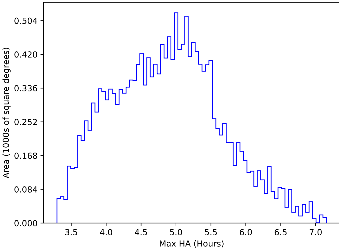
extra_ss_neo4_v3.4_10yrs WFD z band: Max HA
