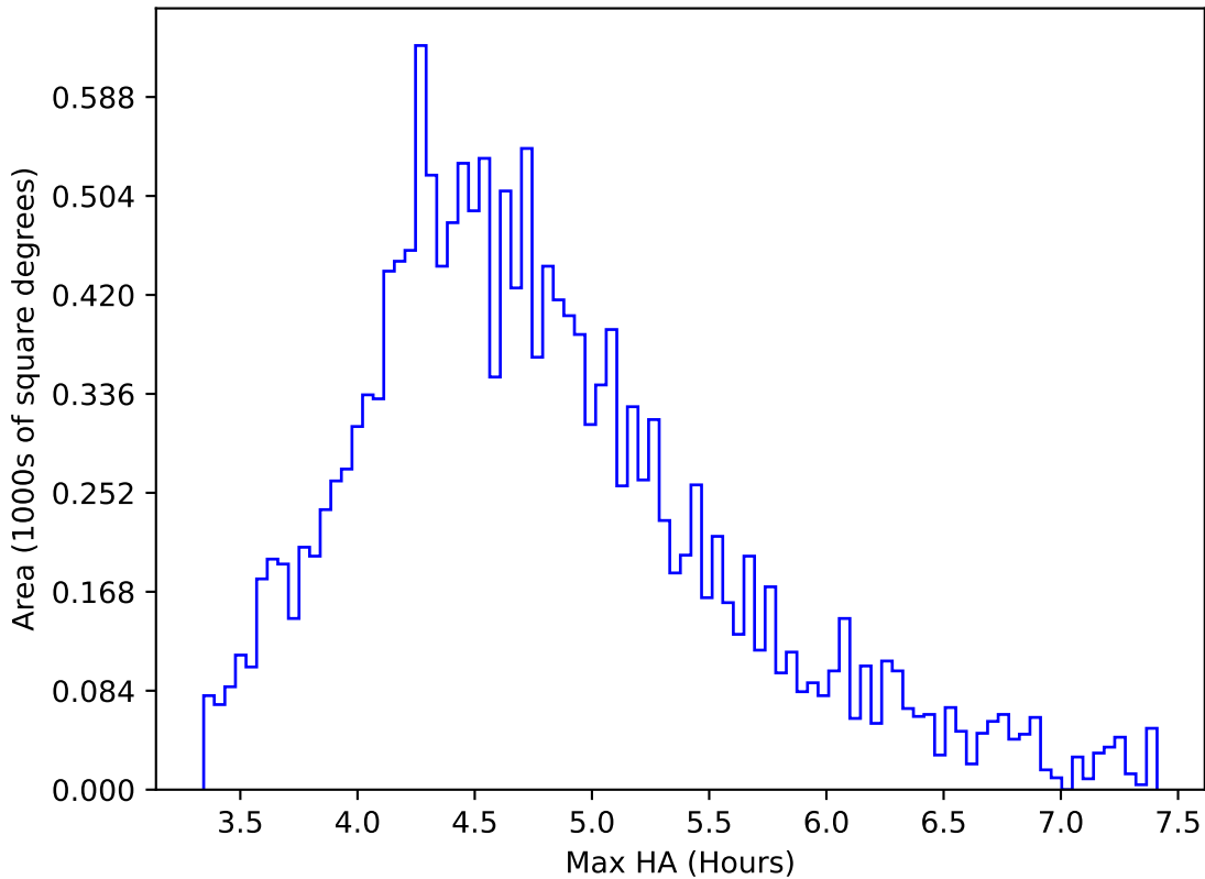
extra_ss_neo4_v3.4_10yrs WFD y band: Max HA
