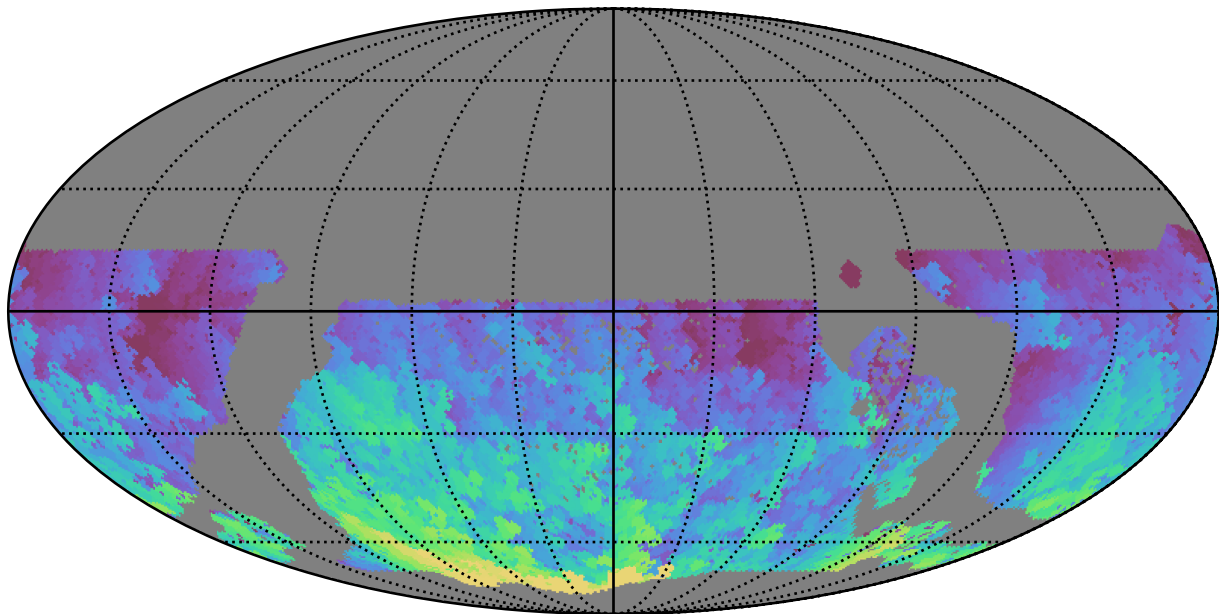
extra_ss_neo4_v3.4_10yrs WFD u band: Max HA
