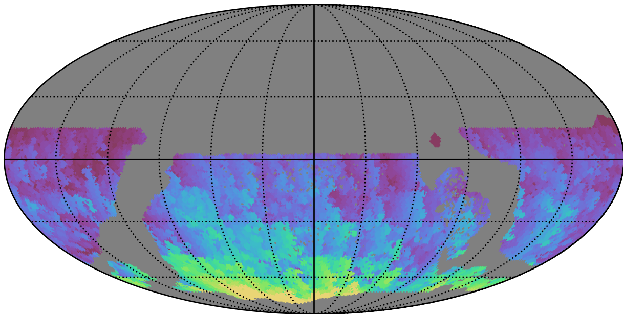
extra_ss_neo4_v3.4_10yrs WFD r band: Max HA
