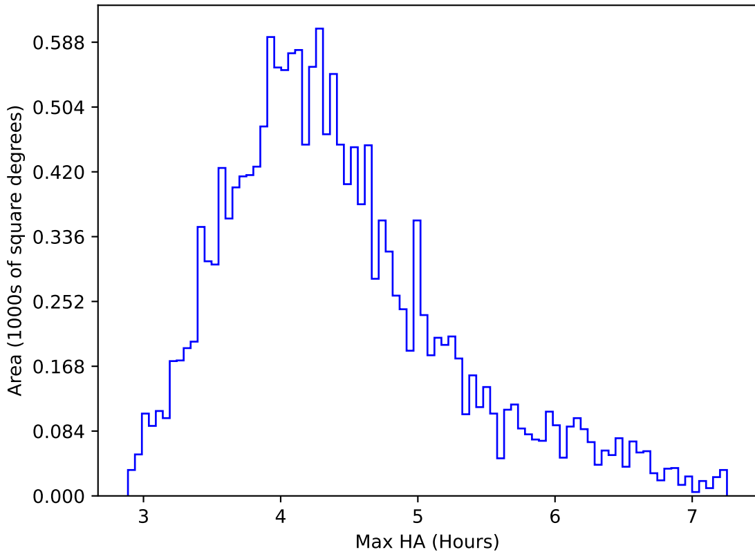
extra_ss_neo4_v3.4_10yrs WFD r band: Max HA
