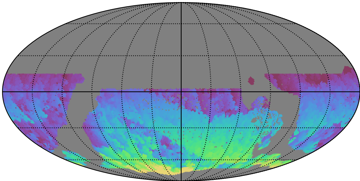
extra_ss_neo4_v3.4_10yrs WFD i band: Max HA
