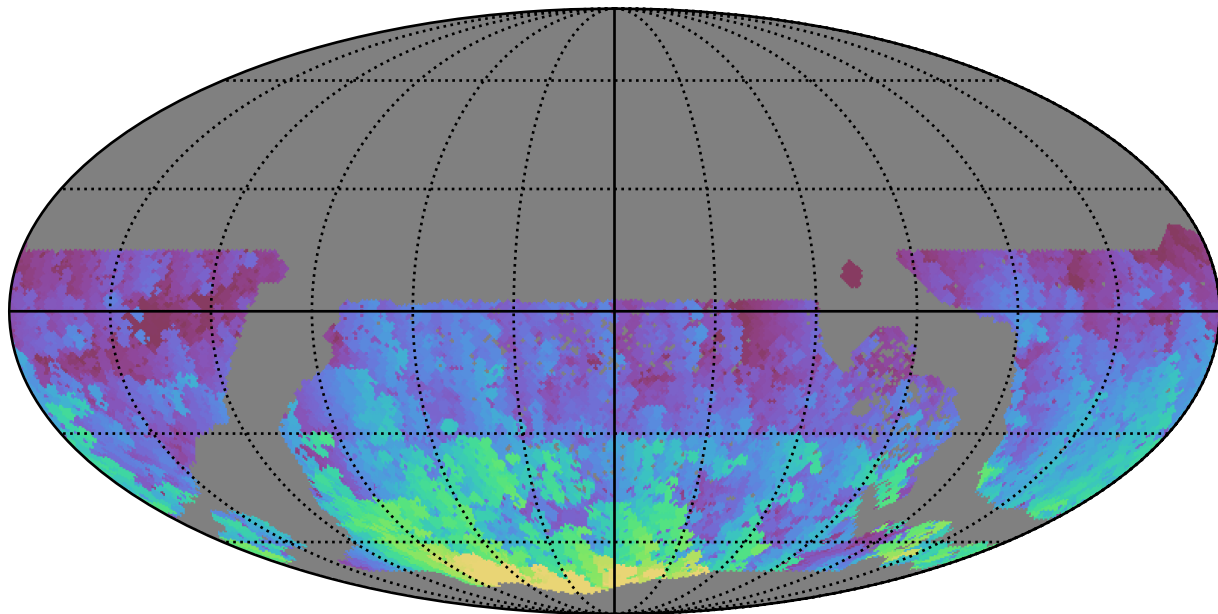
extra_ss_neo4_v3.4_10yrs WFD g band: Max HA
