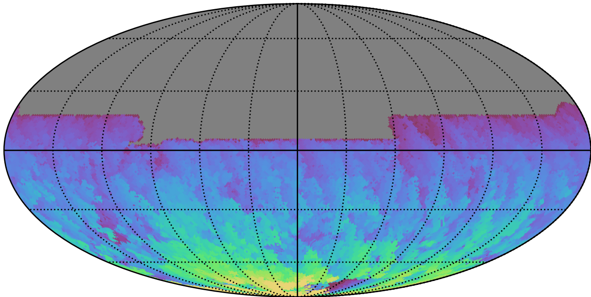
extra_ss_neo4_v3.4_10yrs All sky y band: Max HA
