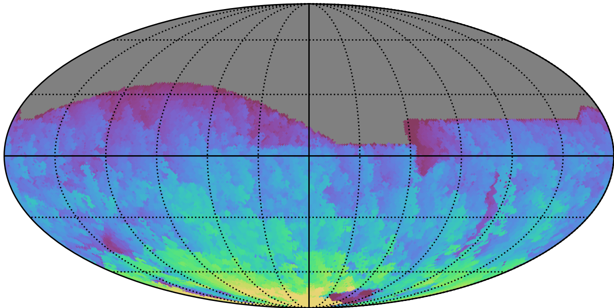
extra_ss_neo4_v3.4_10yrs All sky r band: Max HA
