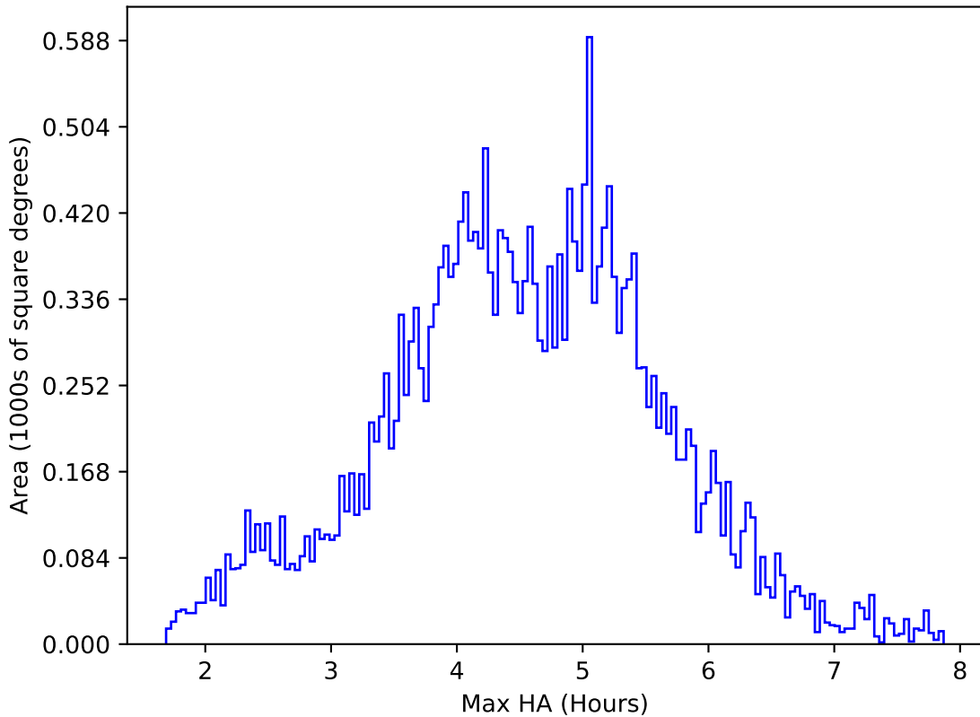
extra_ss_neo4_v3.4_10yrs All sky i band: Max HA
