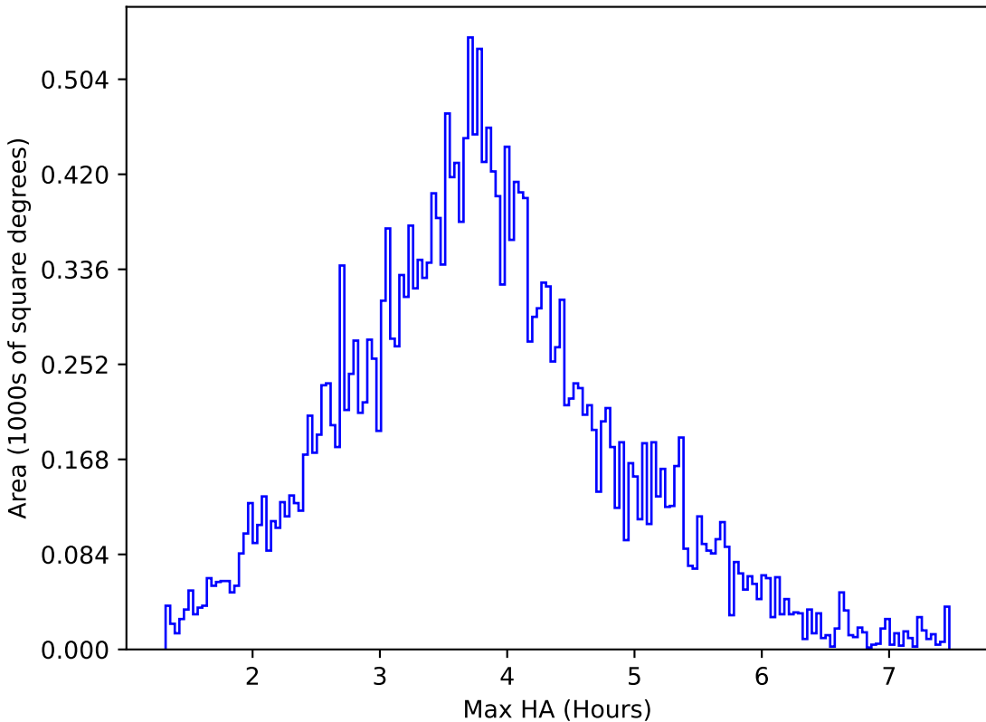
extra_ss_neo4_v3.4_10yrs All sky g band: Max HA
