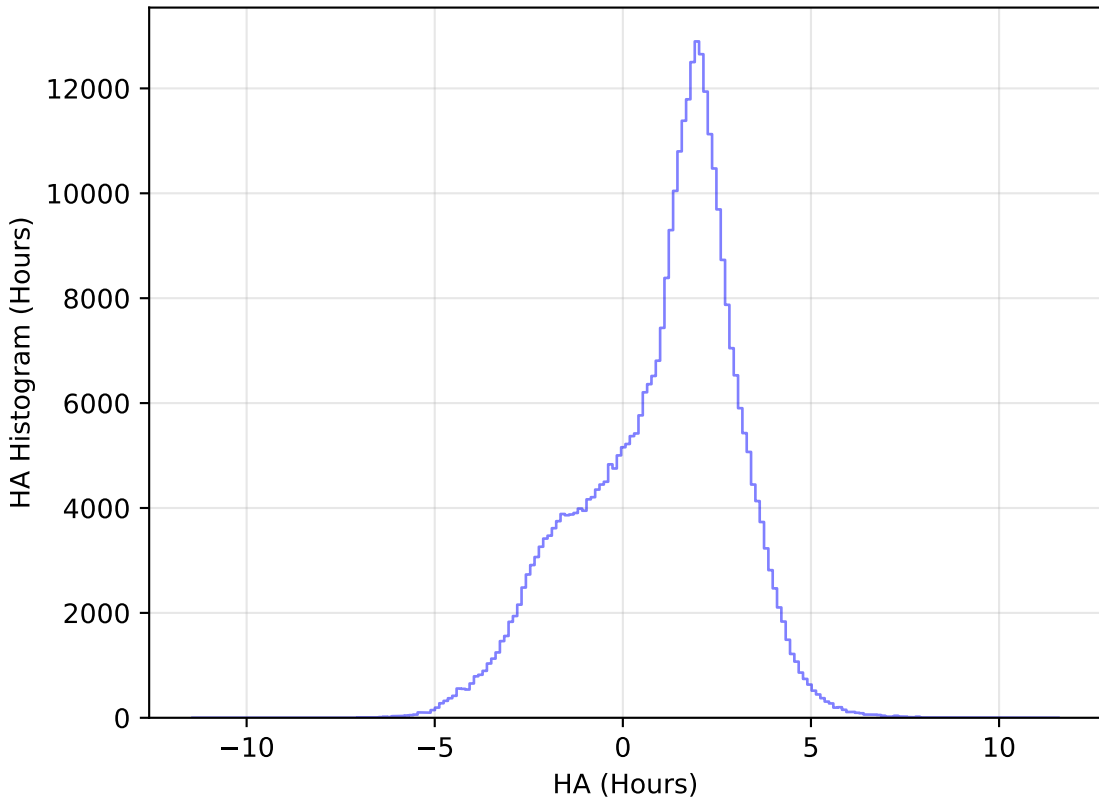
extra_ss_neo4_v3.4_10yrs WFD y band: HA Histogram
