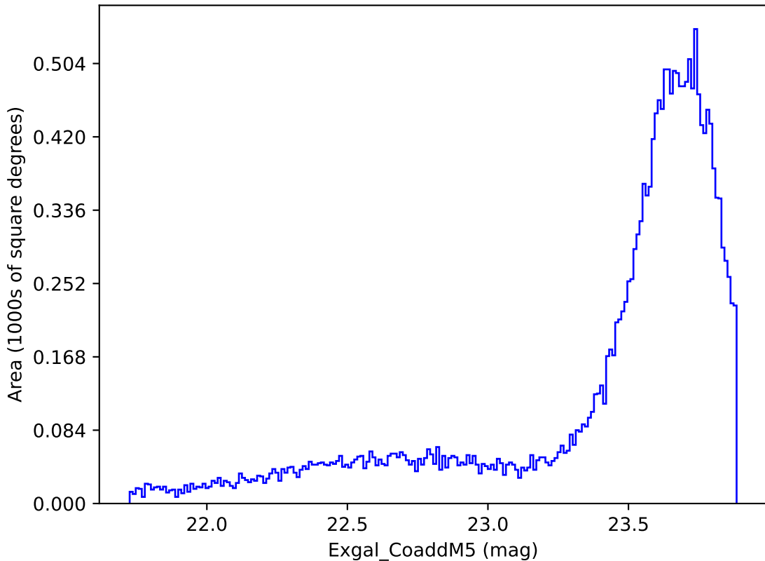
extra_ss_neo4_v3.4_10yrs Yr 1 y band: Exgal_CoaddM5
