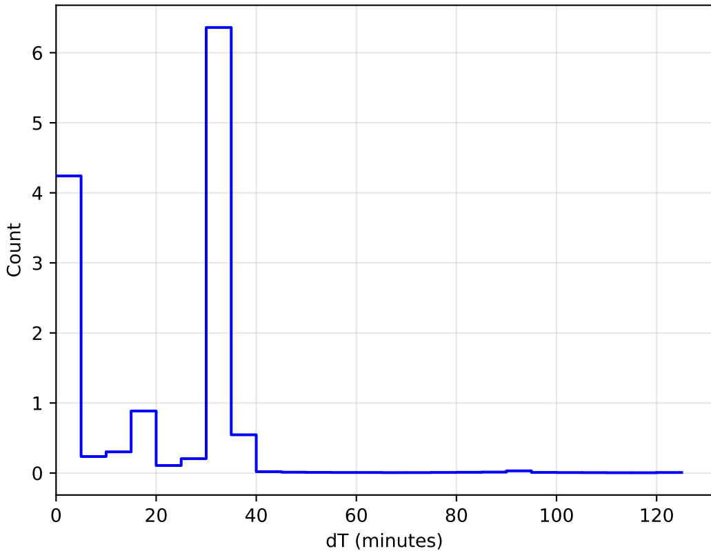
1e6 extra_ss_neo4_v3.4_10yrs All sky: DeltaT Histogram
