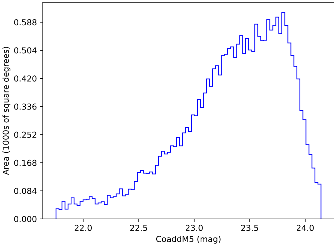
extra_ss_neo4_v3.4_10yrs Yr 3-4 y band: CoaddM5
