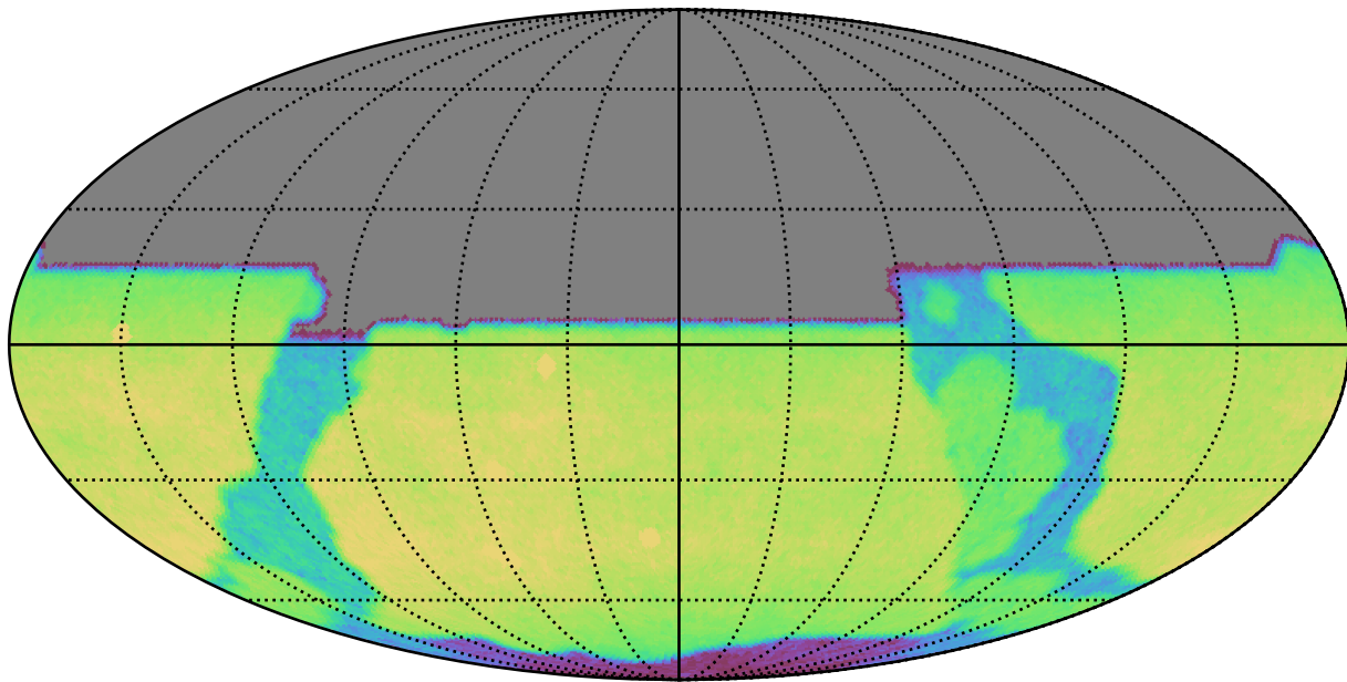
extra_ss_neo4_v3.4_10yrs All sky y band: CoaddM5
