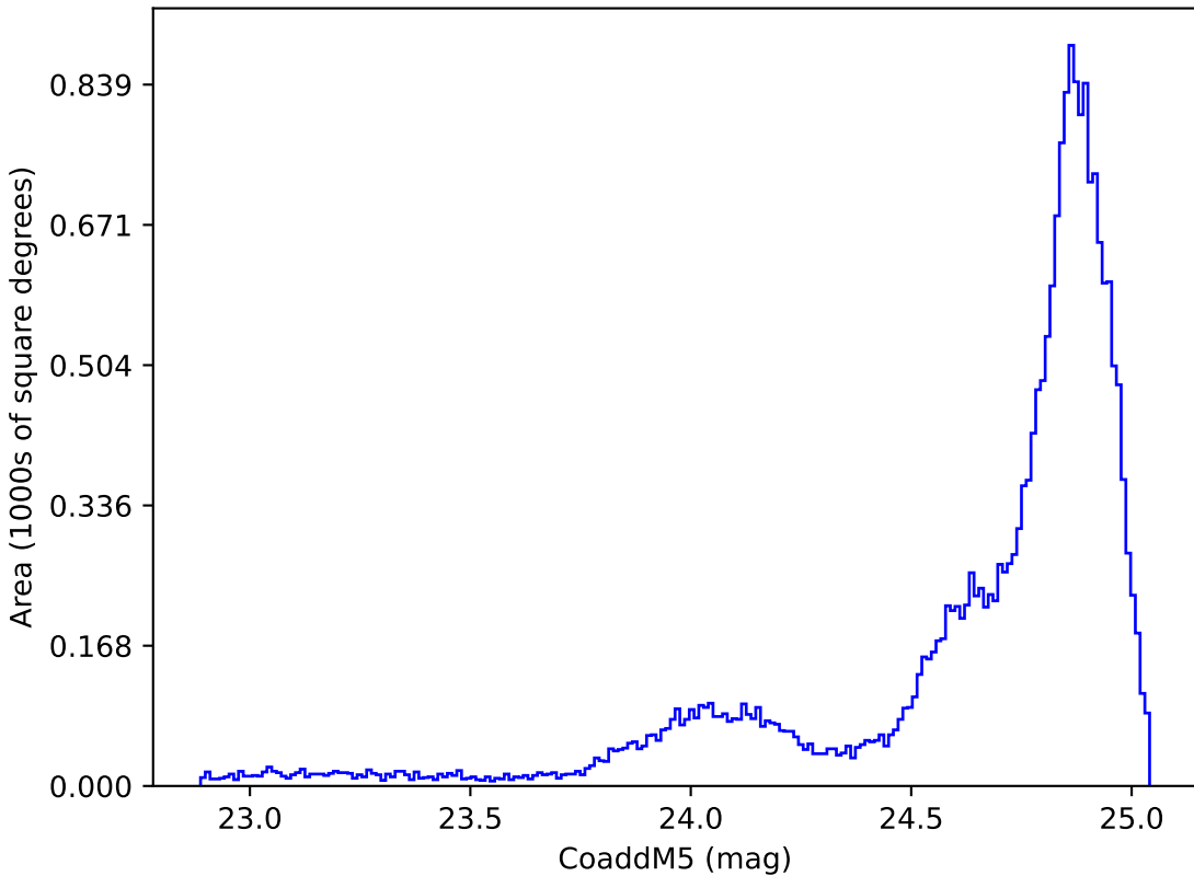
extra_ss_neo4_v3.4_10yrs All sky y band: CoaddM5
