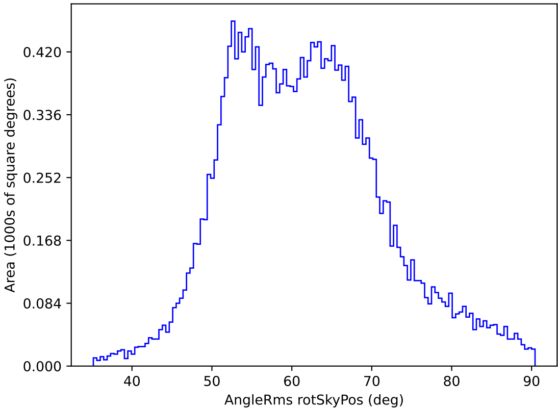
extra_ss_neo4_v3.4_10yrs All sky y band: AngleRms rotSkyPos
