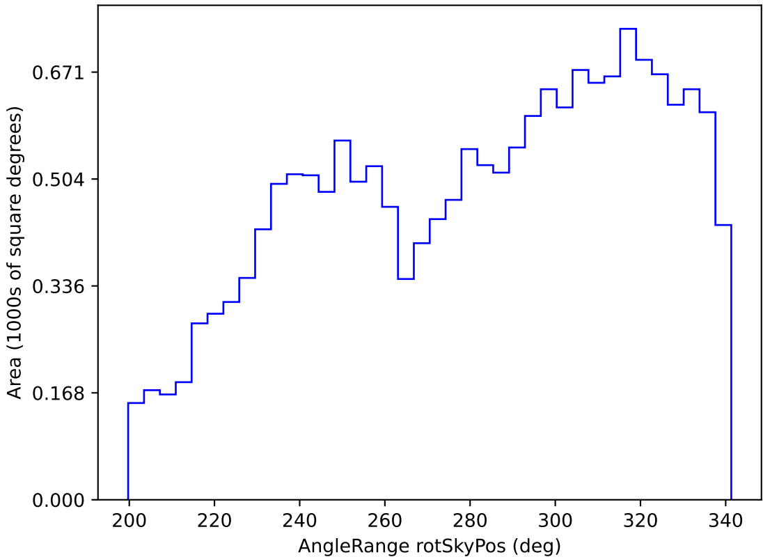
extra_ss_neo4_v3.4_10yrs WFD z band: AngleRange rotSkyPos
