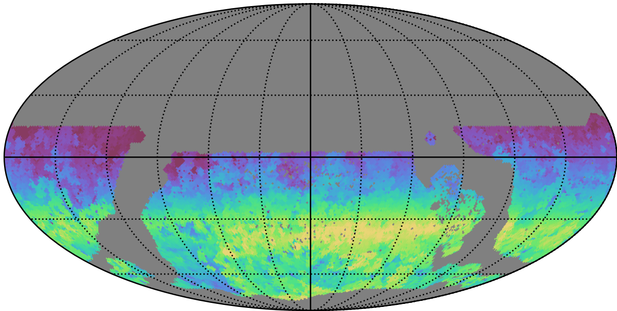
extra_ss_neo4_v3.4_10yrs WFD y band: AngleRange rotSkyPos
