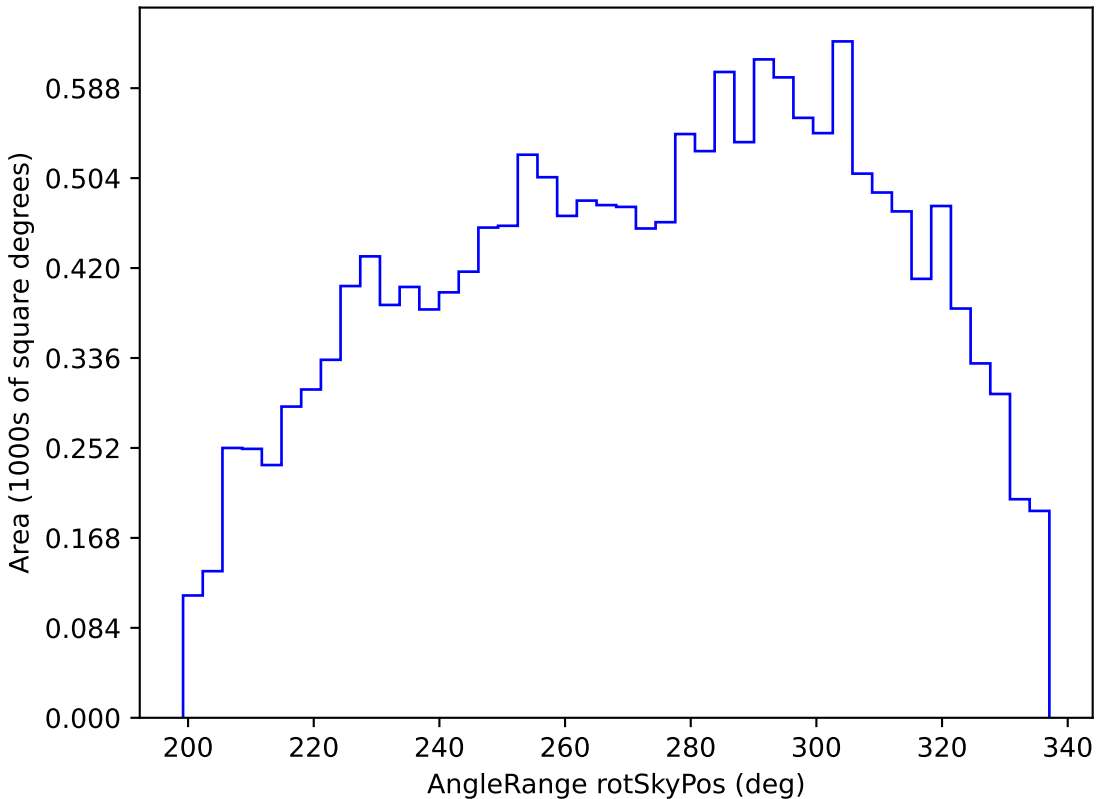
extra_ss_neo4_v3.4_10yrs WFD y band: AngleRange rotSkyPos
