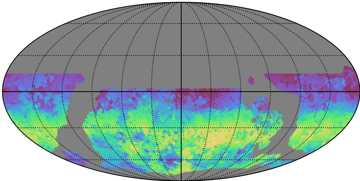
extra_ss_neo4_v3.4_10yrs WFD u band: AngleRange rotSkyPos
