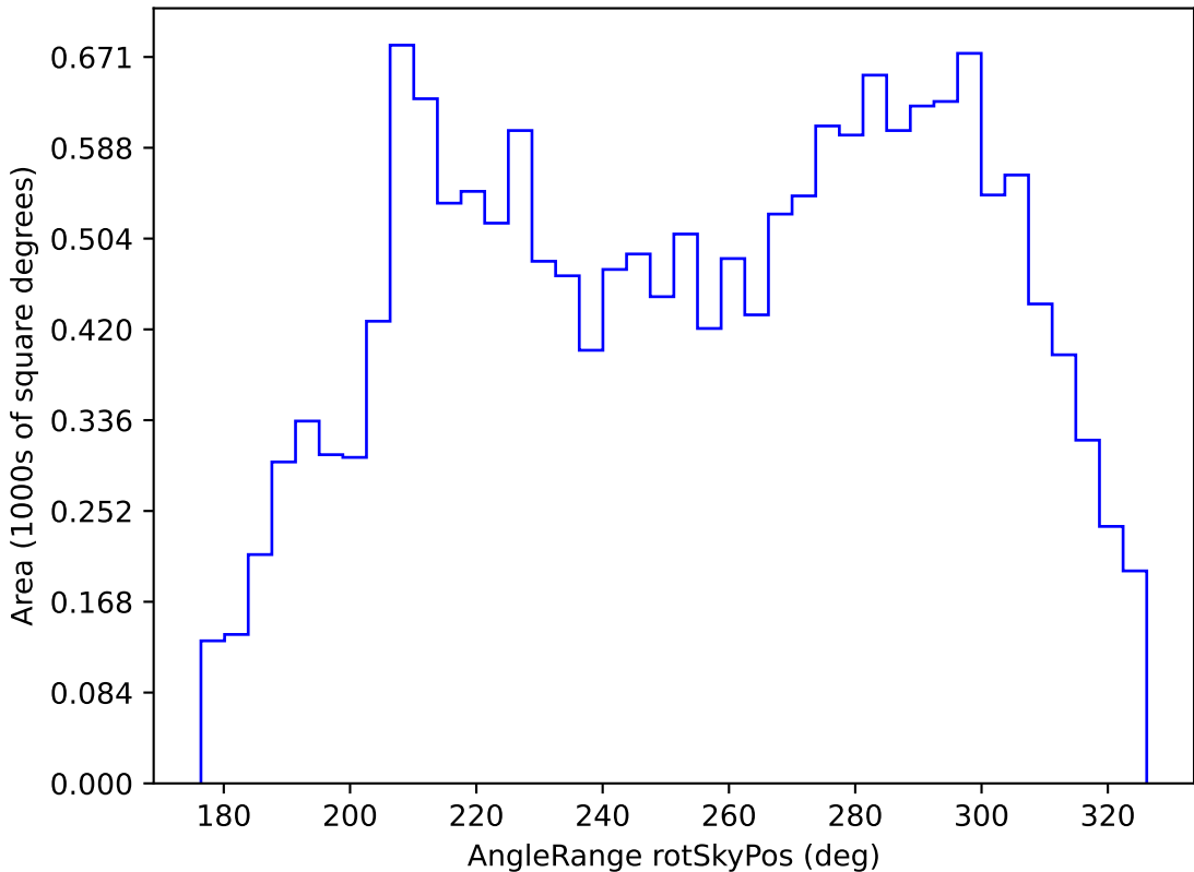
extra_ss_neo4_v3.4_10yrs WFD u band: AngleRange rotSkyPos
