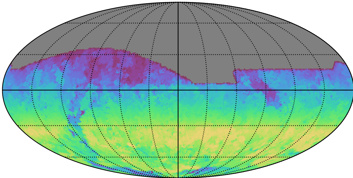
extra_ss_neo4_v3.4_10yrs All sky z band: AngleRange rotSkyPos
