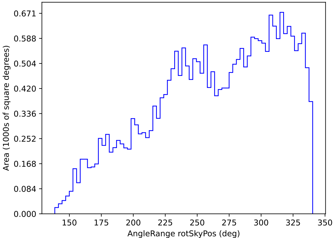
extra_ss_neo4_v3.4_10yrs All sky z band: AngleRange rotSkyPos
